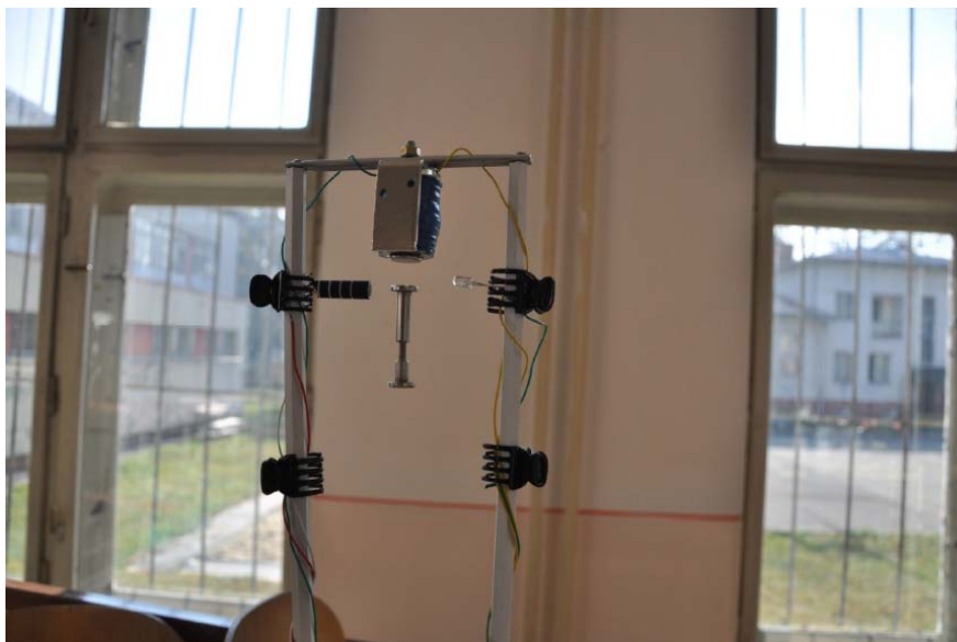
Obr. 1: Elektromagnetický levitátor
