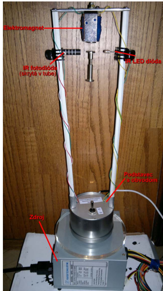
Obr. 1: Elektromagnetický levitátor
